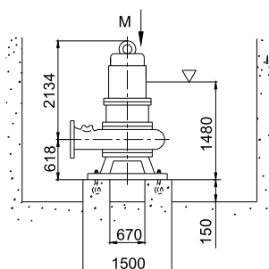
Монтаж на кольцевом основании (P)
