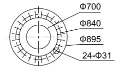
Фланец по стандарту GB/T17241.6PN10
