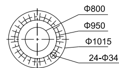
Размер фланца
