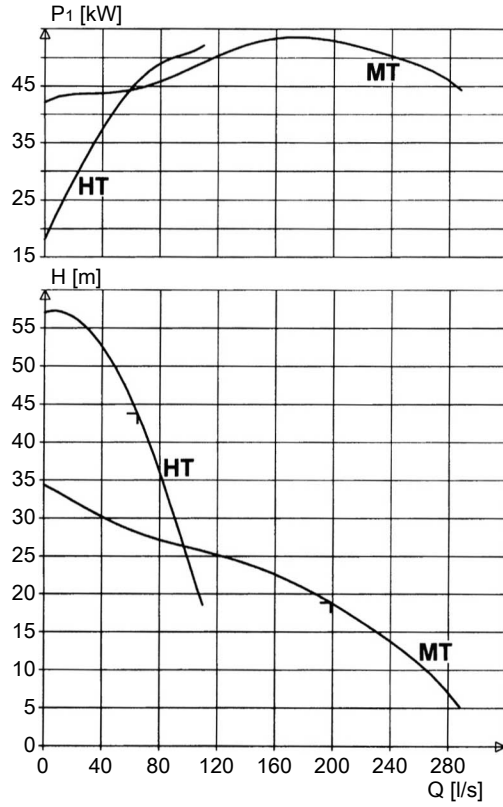
Рис. 7: 50 Гц, 1 470 об/мин
