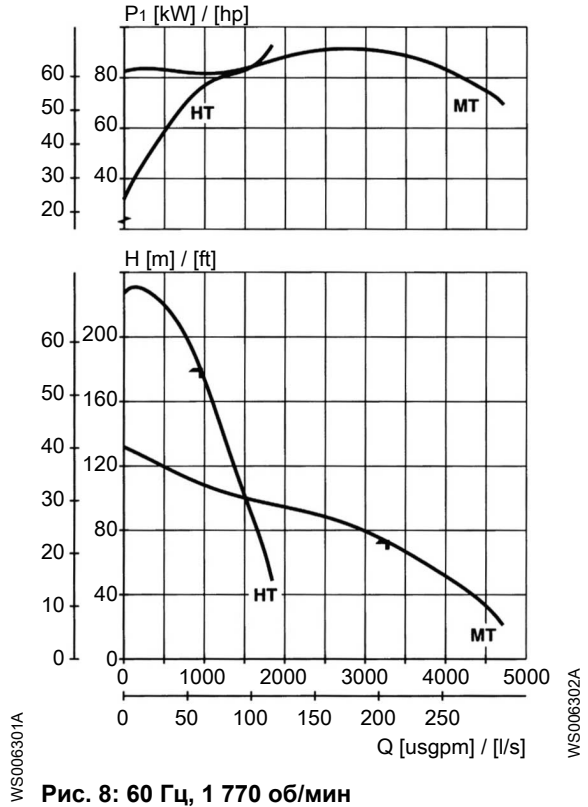
Рис. 8: 60 Гц, 1 770 об/мин
