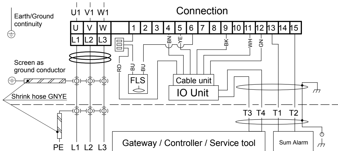
Рис. 8: Невзрывозащищенное исполнение
