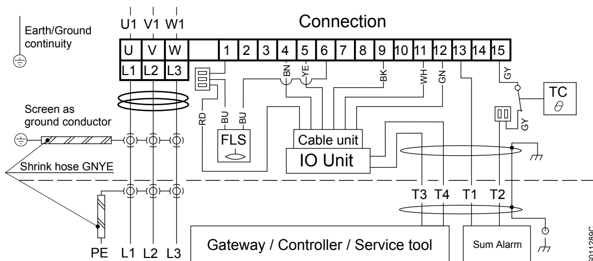
Рис. 9: Взрывозащищенное исполнение
