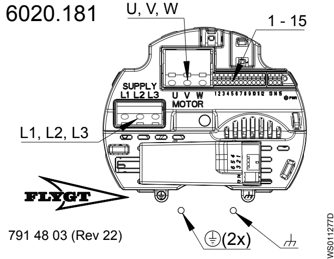
Рис. 6: Невзрывозащищенное исполнение
