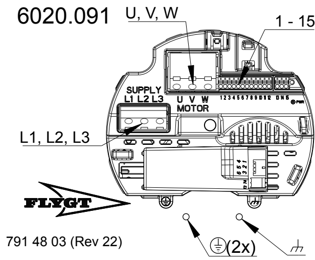
Рис. 7: Взрывозащищенное исполнение
