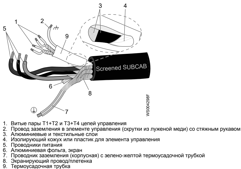
Рис. 3: Подготовленный экранированный SUBCAB™ кабель, без кабельных проушин
