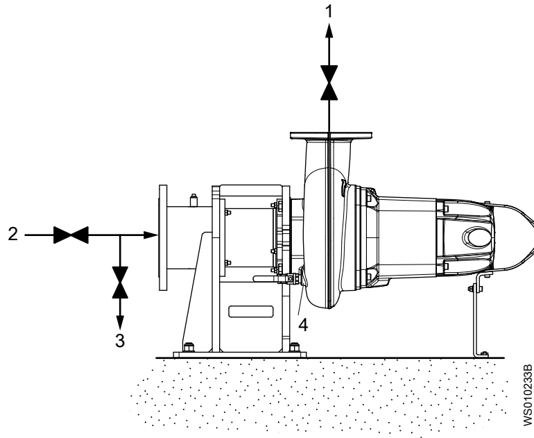
Рис. 12: Установка типа T
