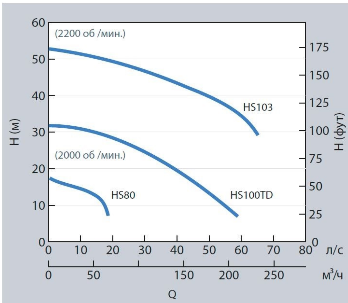
Кривые рабочей характеристики HS80, HS100TD, HS103
